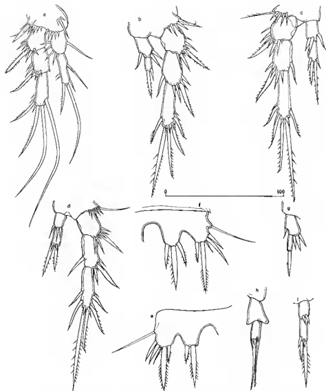
FIG. 6. — Ceuthonectes chappuisi n. sp. a: P 1 ♀; b: P 2 ♀; c: P 3 ♀; d: P 4 ♀; e: P 5 ♂; f: P 5 ♀; g: endopodite P 2 ♂; h: endopodite P 3 ♂; i: endopodite P 4 ♂. (Échelle micrométrique.)
